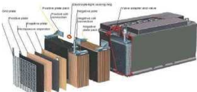
Gambar 3. Konstruksi Baterai
